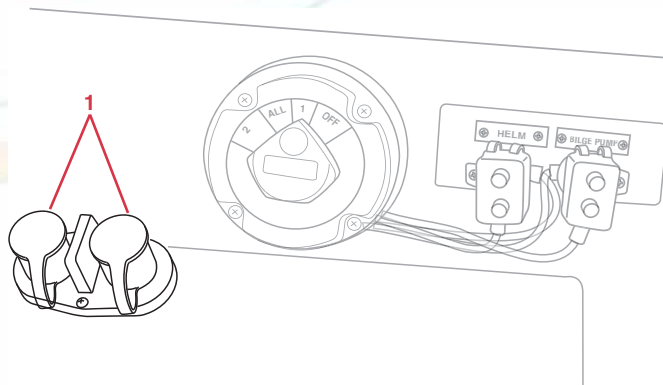
1 – Receptacle
